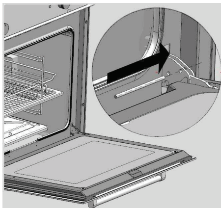
Дверь с наштампованной внутренней рамкой
