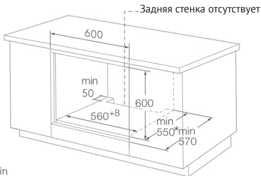
Установка под столешницу
