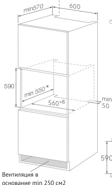
Установка в колонну
